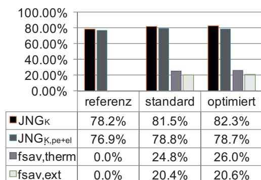
Abbildung 3: Ergebnisse der Jahres-simulationen. JNG K = Kesses-Jahres-nutzungsgrad; JNG K,pe+el = Kessel-Jahres-nutzungsgrad unter miteinbezug der elektrischen Leistung; f sav = fractional energy savings.
